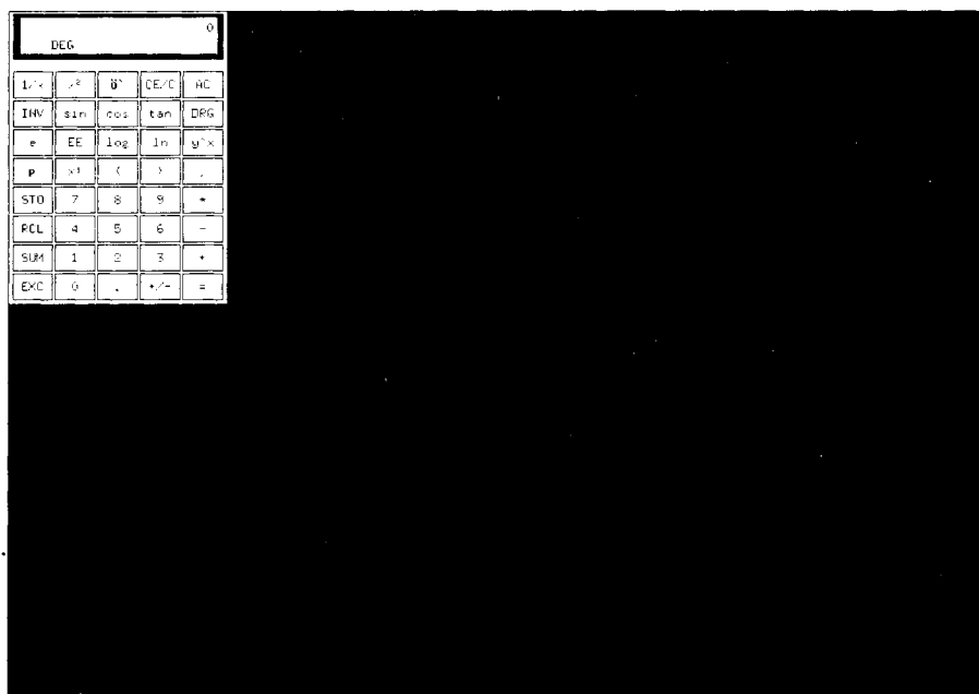
Рис. 16.4. Запуск X-клиента
